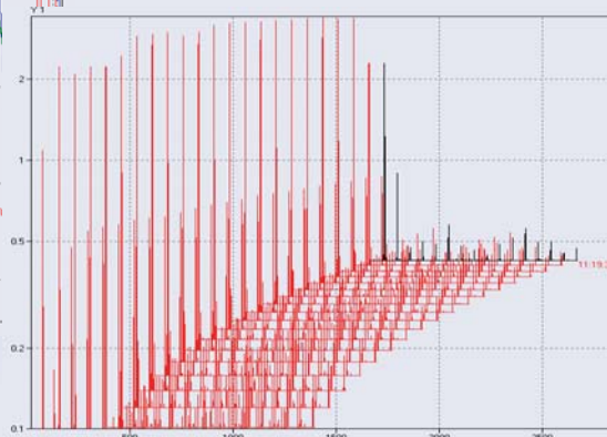
FFT-cascade-diagram
